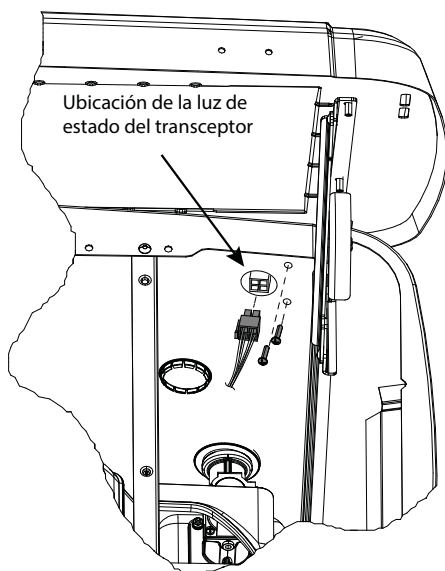
Sujetadores de montaje del transceptor, ubicación de la luz de estado del transceptor y conector de cableado.
